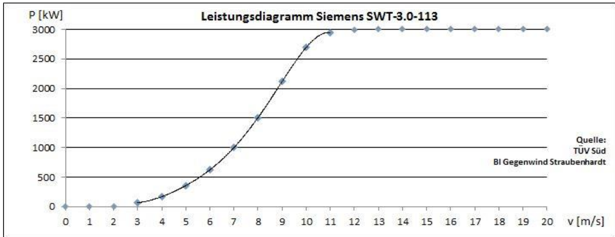
Grafik 2: Kennlinie und Windhäufigkeit in Straubenhardt
