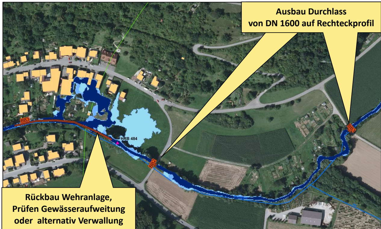
Abbildung 7.5: Vorgeschlagene HWS-Maßnahmen Ortseingang Stein, Sandgrube
