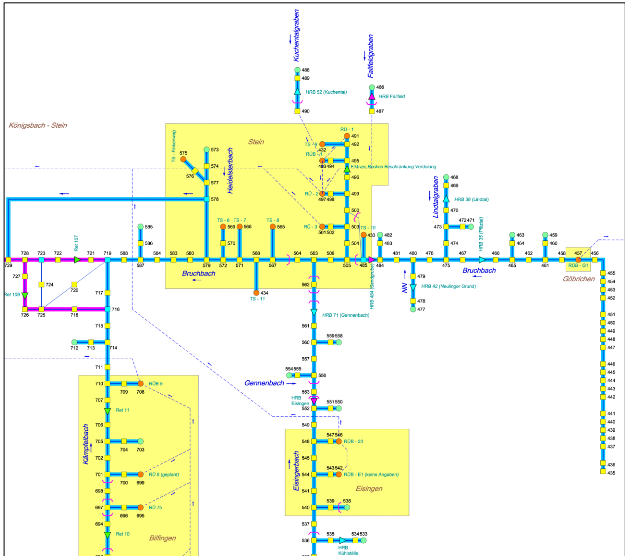
Abbildung 1.6: FGM-Pfingtal - Ausschnitt der Systemskizze für den Bereich der FGU-Stein (Bruchbach)
