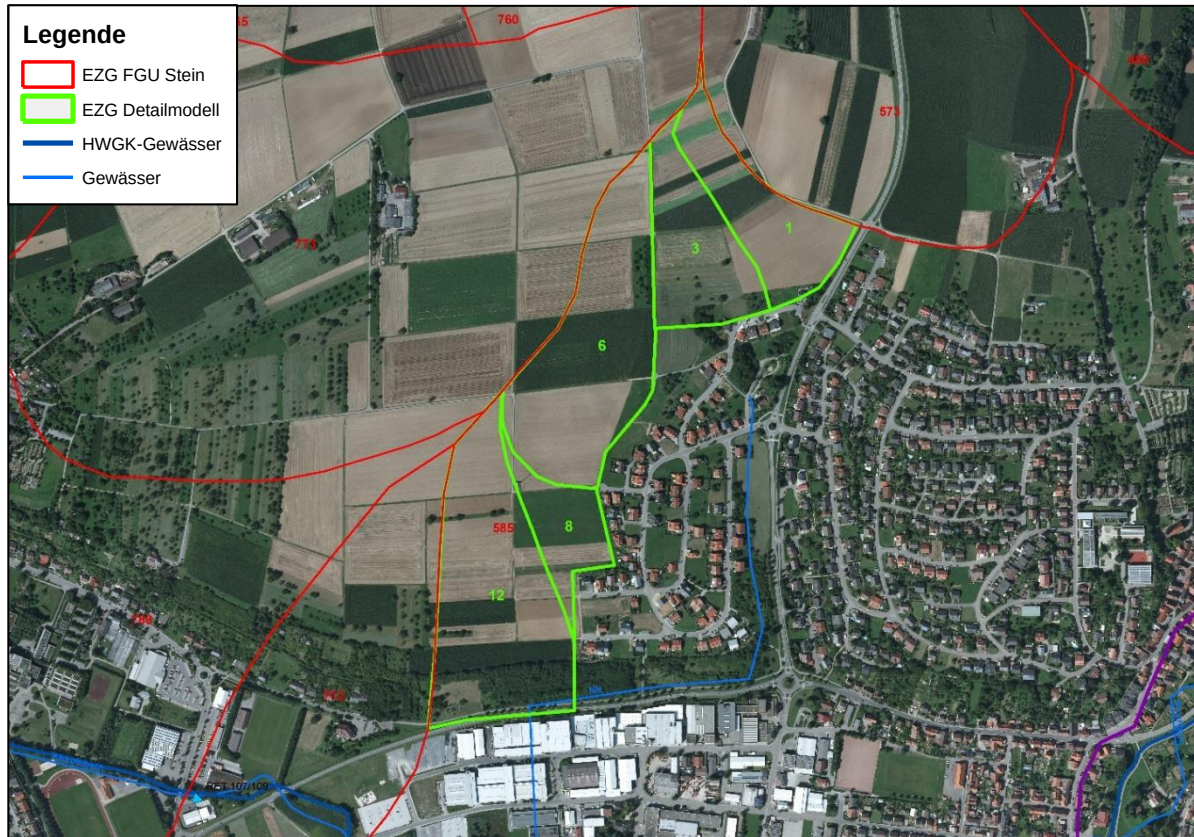
Abbildung 7.24: Räumliche Gliederung des FGM-Detailmodells Königsbacher Berg
