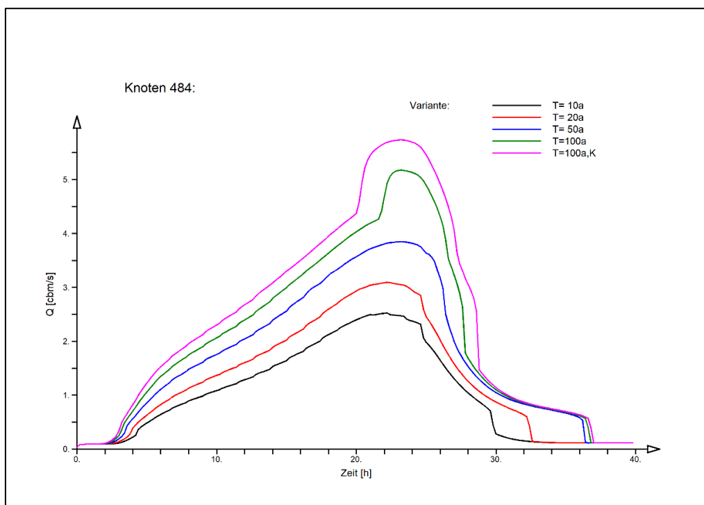
Abbildung 4.21: Bruchbach im Bereich Ortseingang Stein, Sandgrube, HW-Ganglinien T_D=24h der FGM-Var. „IO“ (Ist-Zustand) für Ereignisse unterschiedlicher Jährlichkeiten T
