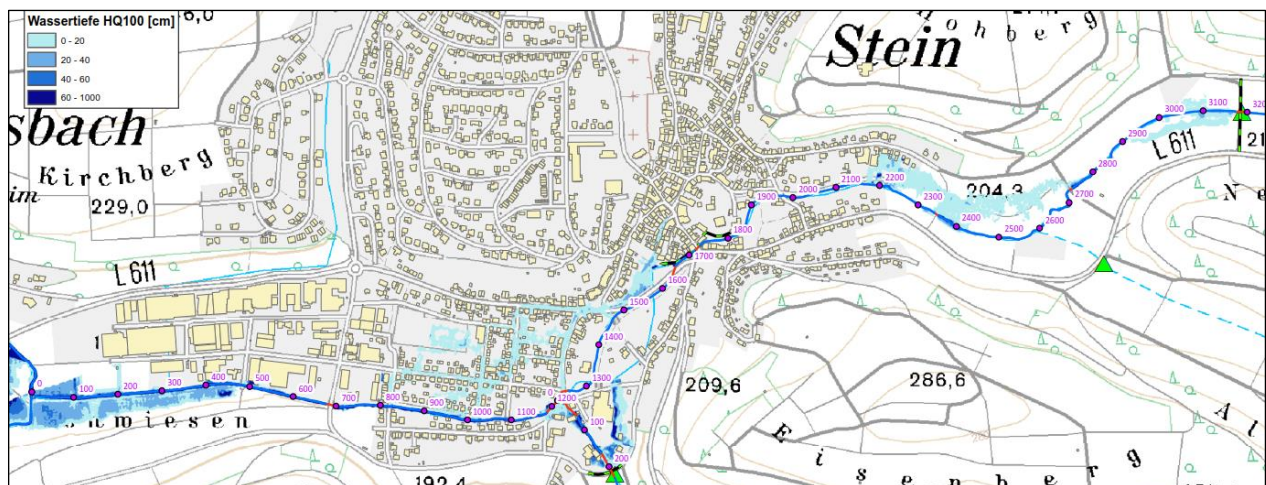
Abbildung 5.7: Teilbereich Bruch-, Gennenbach – Wassertiefenkarte (100a) für den Ist-Zustand
