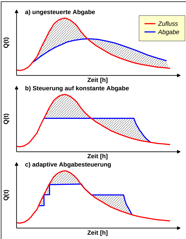
Abbildung 4.1: Abgabearten von Hochwasserrückhaltebecken (nach Ihringer, 2005)
