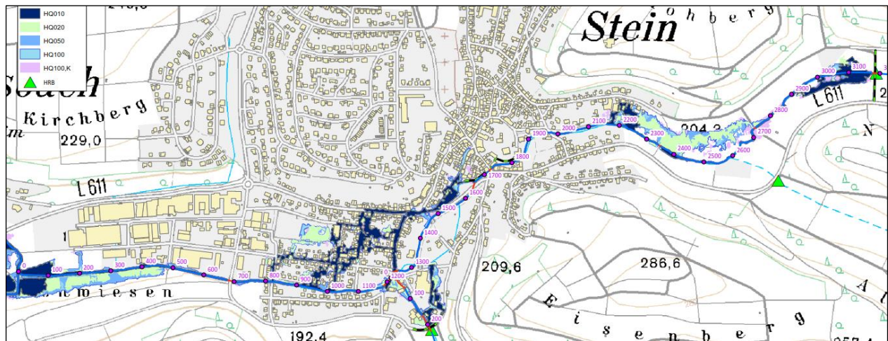
Abbildung 5.6: Teilbereich Bruch-, Gennenbach – Überflutungskarte (10a,20a,50a,100a, 100aKlima) für den Ist-Zustand
