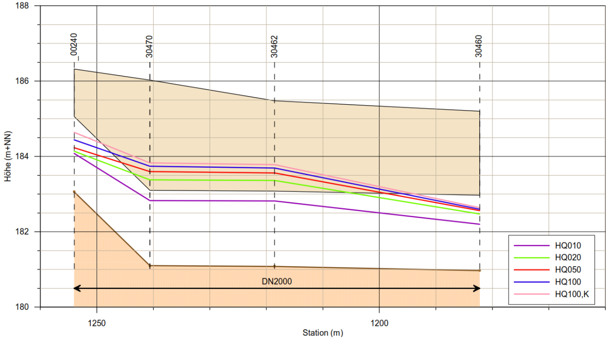
Abbildung 5.9: Längsschnitt Verdolung Bruchbach, WSP-Lagen HQ10, HQ20, HQ50, HQ100, HQ100K
