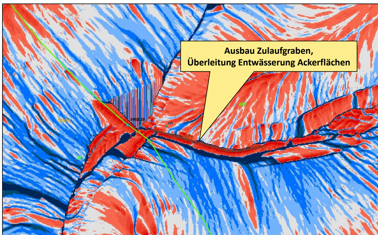
Abbildung 7.3: Fließwegberechnung Bereich Lindtal mit vorgeschlagener HWS-Maßnahme LT1
