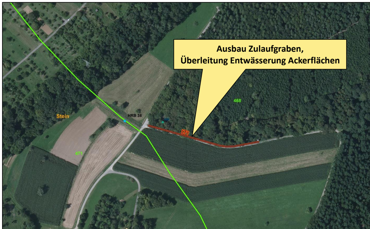
Abbildung 7.2: Lageplan HRB-38 Lindtal mit vorgeschlagener HWS-Maßnahme LT1
