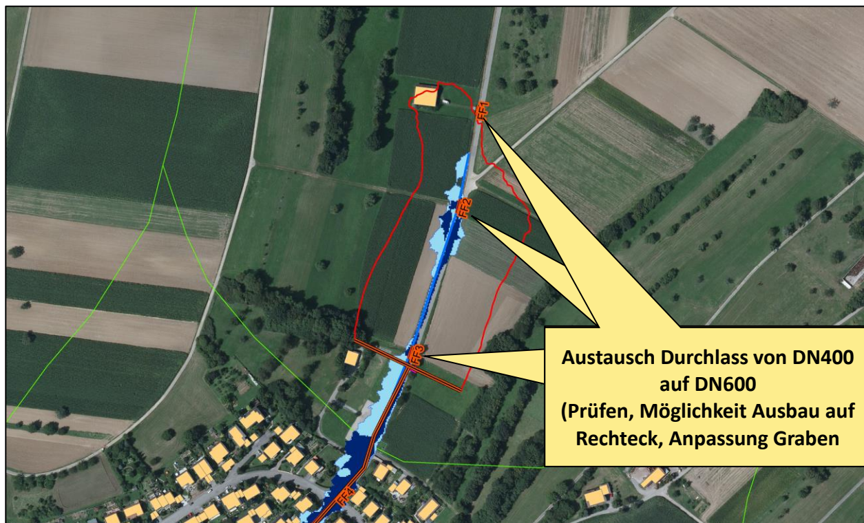
Abbildung 7.17: Vorgeschlagene lokale HWS-Maßnahmen Fallfeld (vor der Ortslage)
