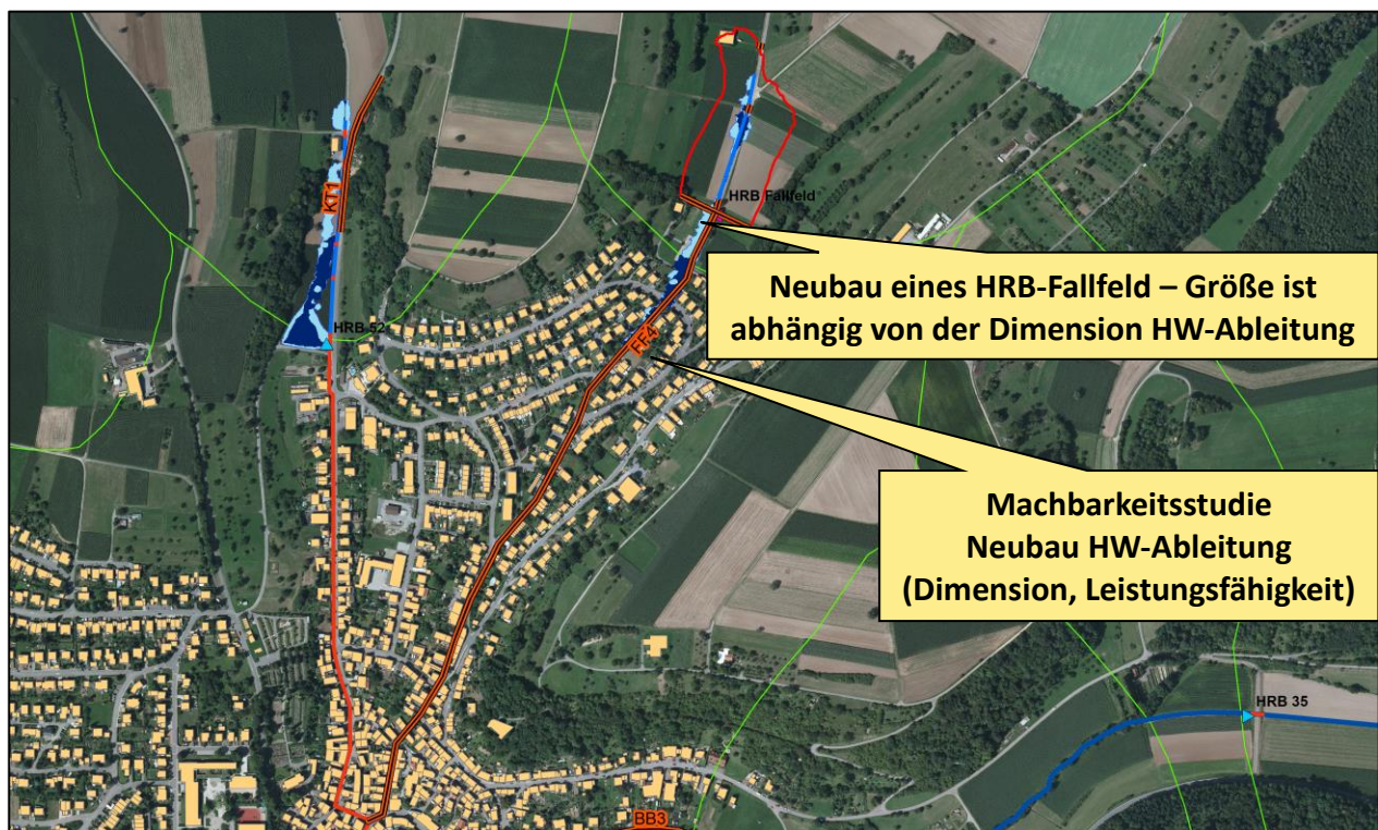
Abbildung 7.18: Mögliche HWS-Maßnahmen Fallfeld, Machbarkeitsstudie HRB Fallfeld und HW-Ableitung
