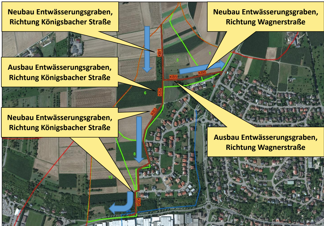
Abbildung 7.26: Vorgeschlagene HWS-Maßnahmen Detailmodell Königsbacher Berg
