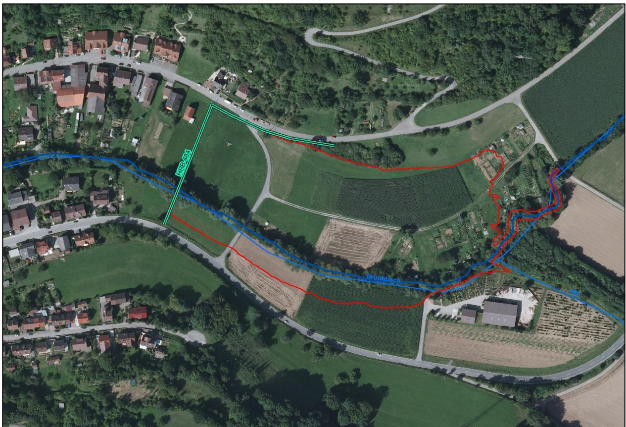
Abbildung 4.14: Mögliches HRB-484 Bruchbach – Lageskizze
