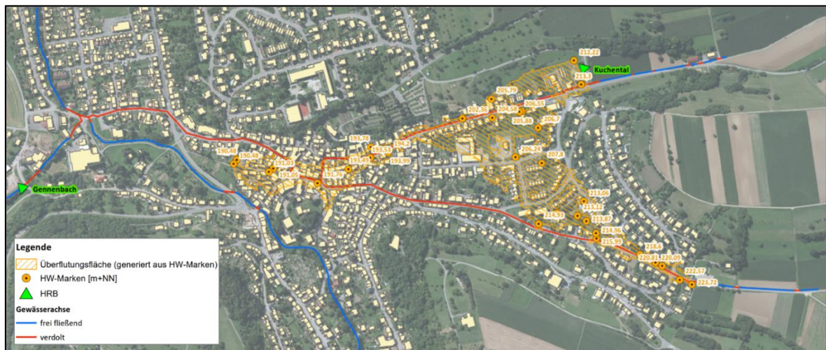
Abbildung 6.5: Kuchental-, Fallfeldgraben, HW-Marken und daraus generierte Überflutungsfläche des HW-Ereignisses 2016
