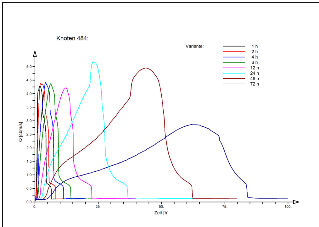
Abbildung 4.20: Bruchbach im Bereich Ortseingang Stein, Sandgrube, HW-Ganglinien T=100a der FGM-Var. „IO“ (Ist-Zustand) für Ereignisse unterschiedlicher Regendauern T_D
