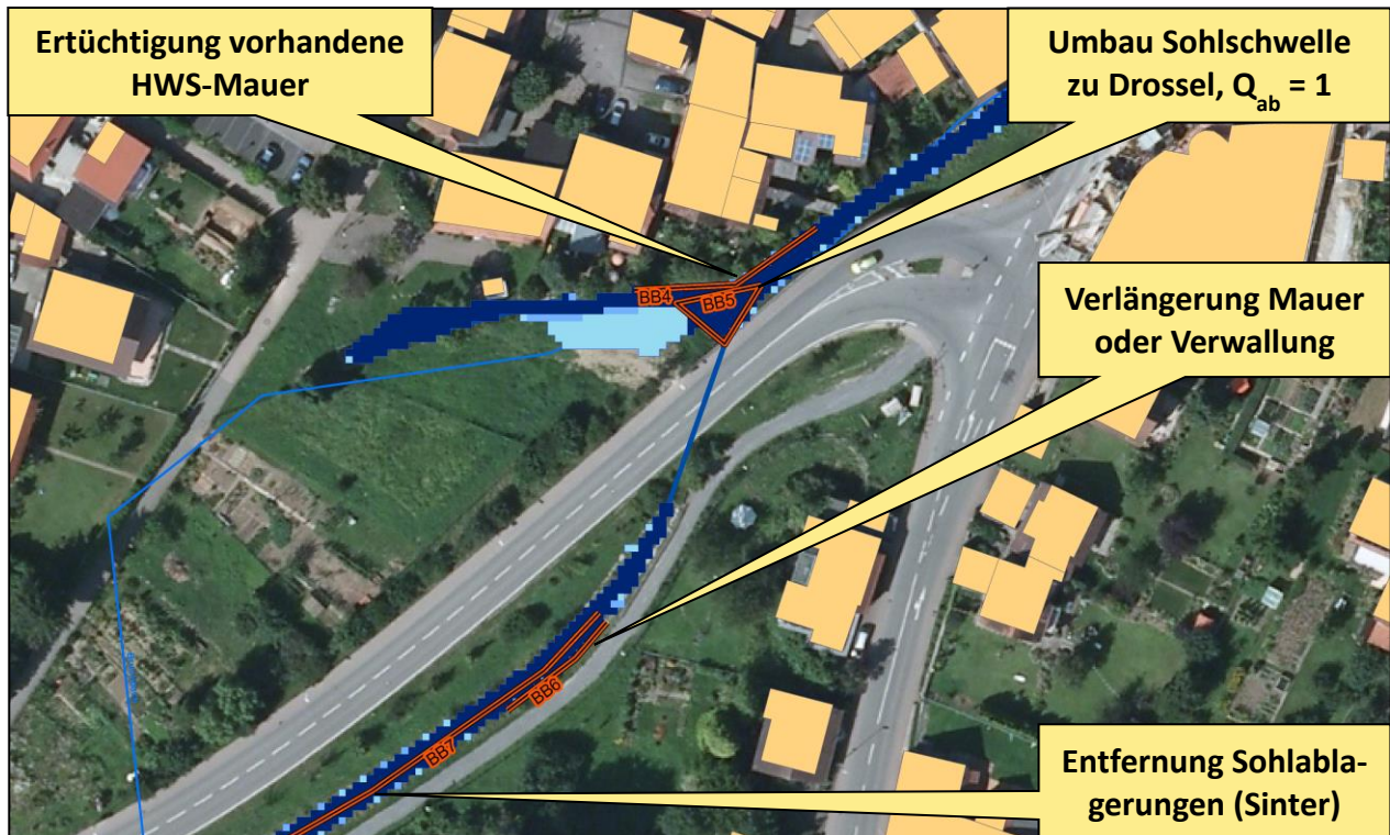
Abbildung 7.9: Vorgeschlagene HWS-Maßnahmen Stein Zentrum, Querung L611
