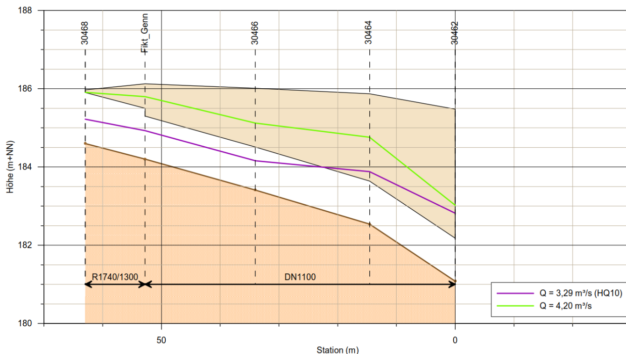
Abbildung 5.10: Längsschnitt Verdolung Gennenbach, WSP-Lagen
