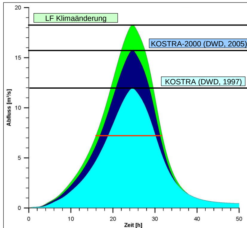
Abbildung 3.5: Vergleich von FGM-Berechnungen (fiktives Testgebiet) aus KOSTRA (DWD, 1997), KOSTRA-2000 (DWD, 2005/2009) und LF Klimaänderung
