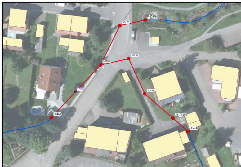
Abbildung 5.8: Detailausschnitt Verdolung Mündungsbereich Bruch-, Gennenbach
