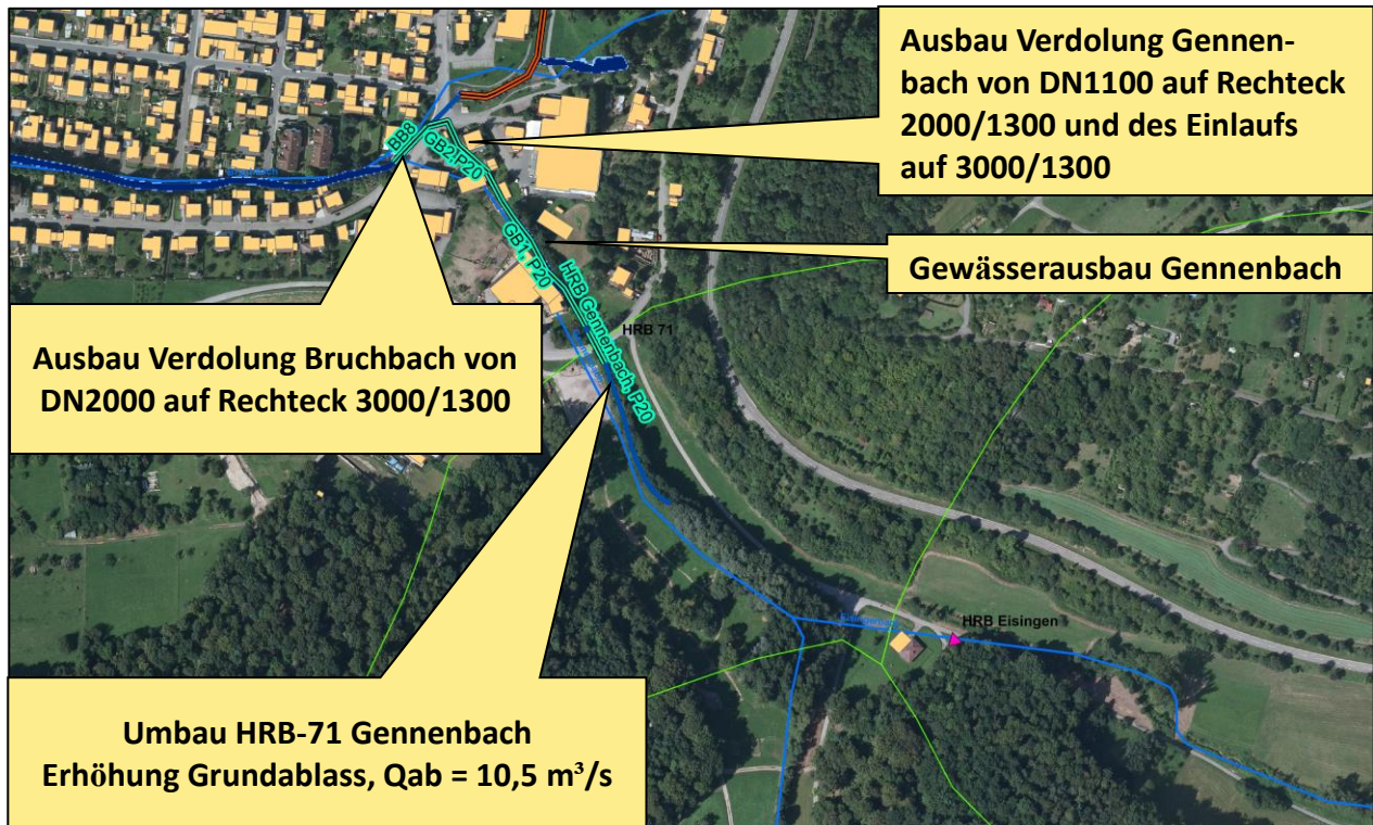
Abbildung 8.1: Untersuchte HWS-Maßnahmen „P20“ (verworfen) am Gennenbach
