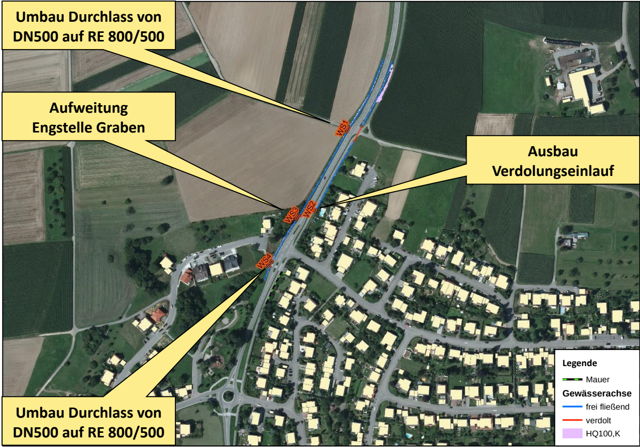
Abbildung 7.21: Vorgeschlagene HWS-Maßnahmen Heidelsterbach
