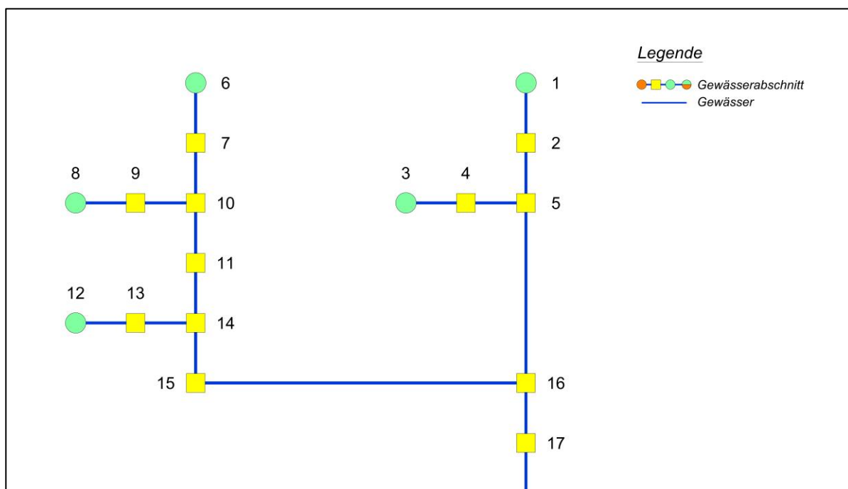
Abbildung 7.25: Systemskizze des FGM-Detailmodells Königsbacher Berg
