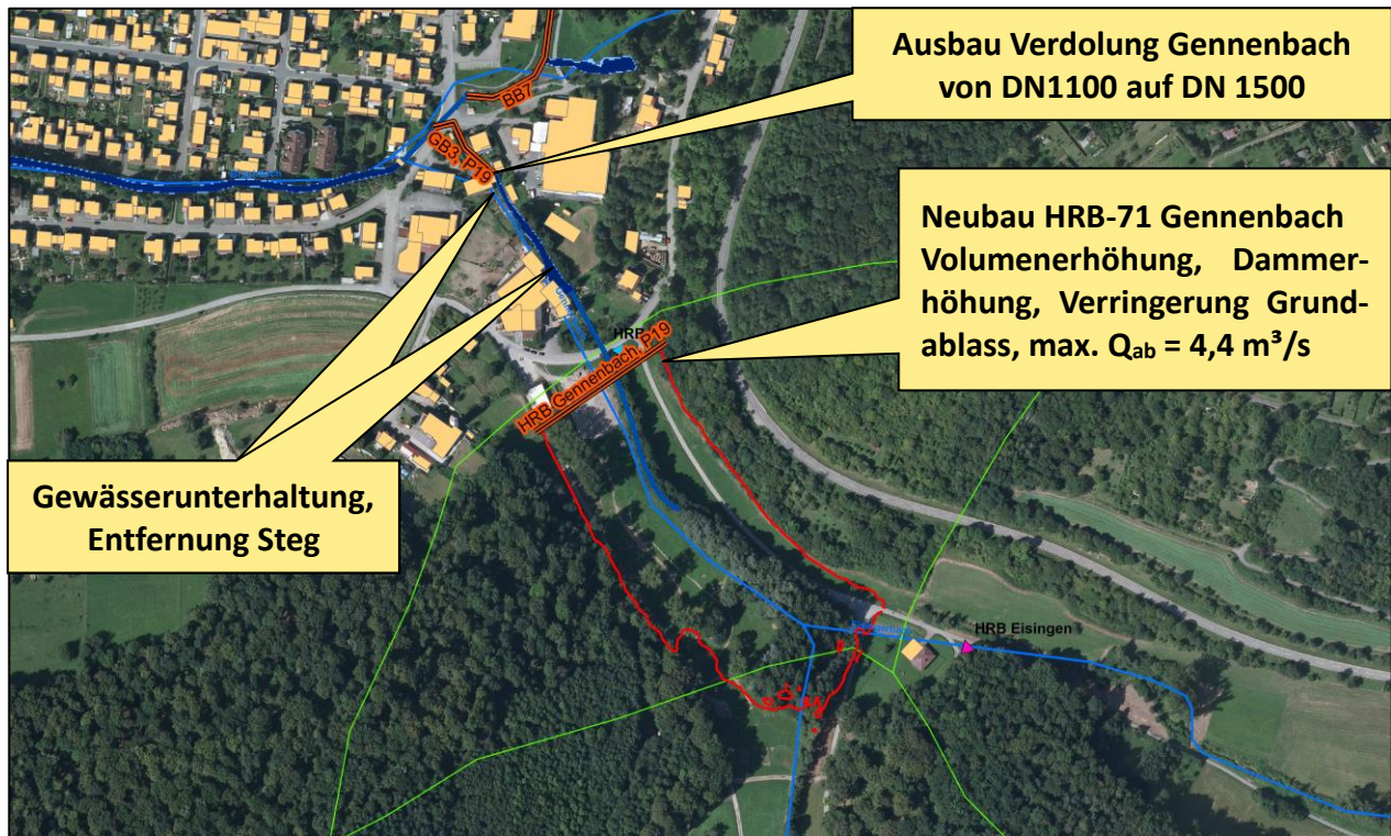
Abbildung 7.15: Vorgeschlagene HWS-Maßnahmen Gennenbach
