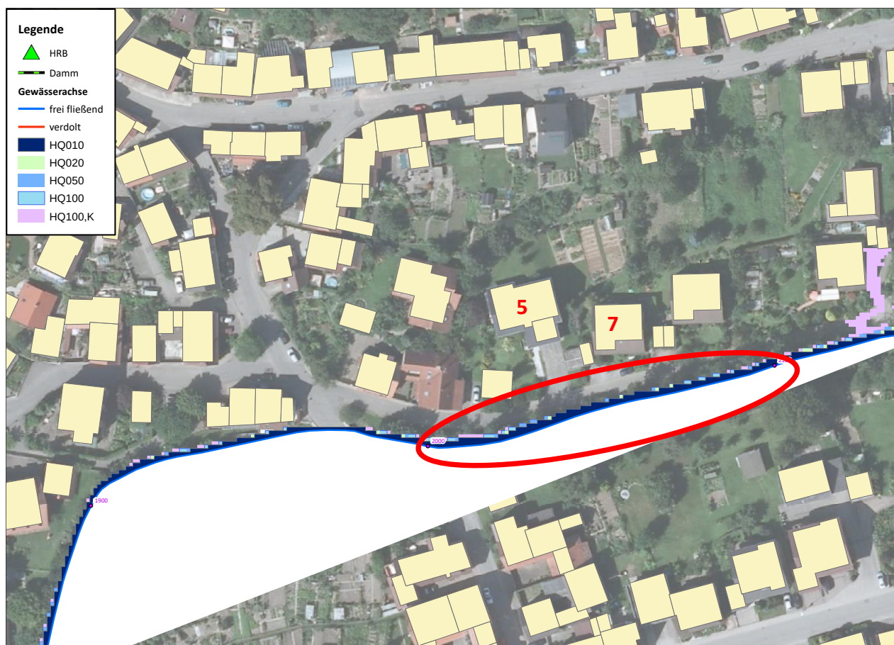
Abbildung 8.5: Beschriebene Schwachstelle am Bruchbach, „Sandgrube 5 - 7“
