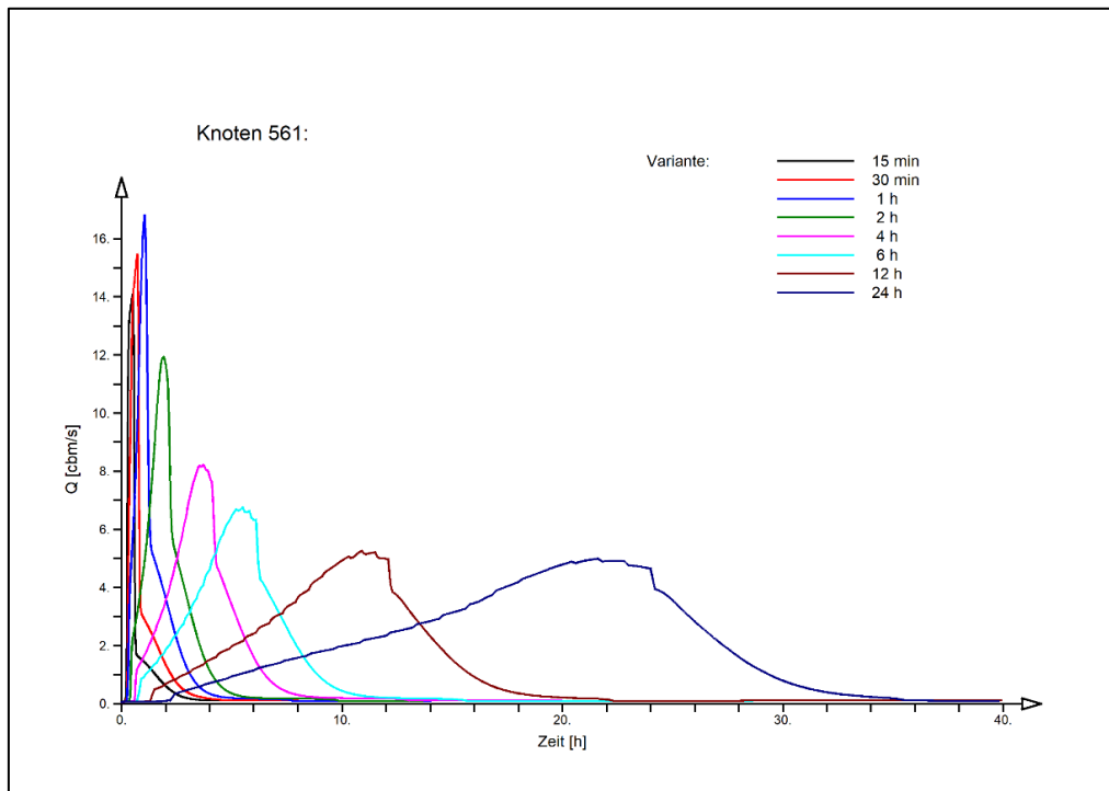
Abbildung 4.22: Gennenbach Zulauf HRB Gennenbach, HW-Ganglinien T=100a der FGM-Var. „I0“ (Ist-Zustand) für Ereignisse unterschiedlicher Regendauern T_D
