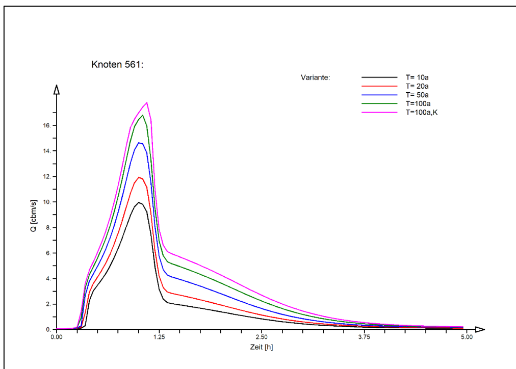
Abbildung 4.23: Gennenbach Zulauf HRB Gennenbach, HW-Ganglinien T_D=1h der FGM-Var. „I0“ (Ist-Zustand) für Ereignisse unterschiedlicher Jährlichkeiten T
